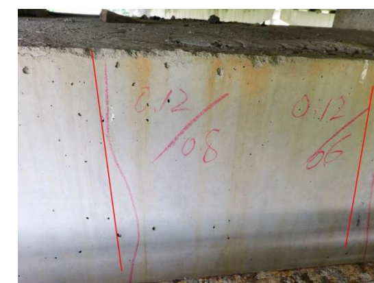
图 3-10：九湖分离（下行）GL-20D 盖梁：距左侧 1m 处，小桩号面竖向裂缝；数量：2 条，长度：0.7m，宽度：0.12mm。
