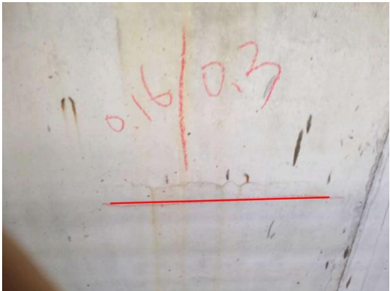
图 3-12: 建华村大桥(上行) GL-4D 盖梁: 距左侧 2m 处, 距上缘 0.4m 处, 大桩号面横向裂缝; 数量: 1 条, 长度: 0.3m, 宽度: 0.16mm。
