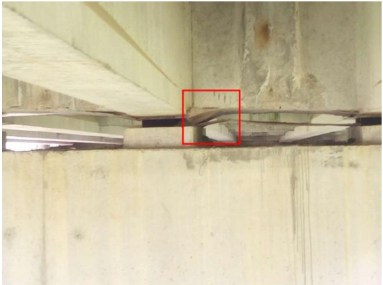
图 3-17: 建华村大桥(下行) ZZ-2-1-4 支座: 混凝土包裹; 数量: 1 个。
