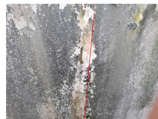
图 3-9：草板大桥（下行）GL-8D 盖梁：距左侧 2m 处，距上缘 0m 处，大桩号面竖向裂缝；数量：1 条，长度：1m，宽度：0.14mm。
